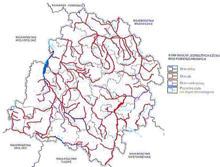
Rys. 7. Jakość wód powierzchniowych w województwie łódzkim
