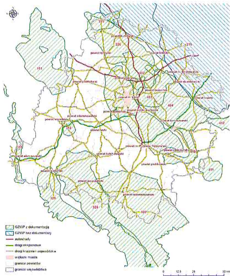
Mapa 2. Lokalizacja GZWP na terenie województwa łódzkiego
