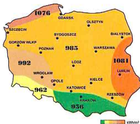
Rys.6. Podział Polski ze względu na rozkład sum rocznego promieniowania słonecznego
