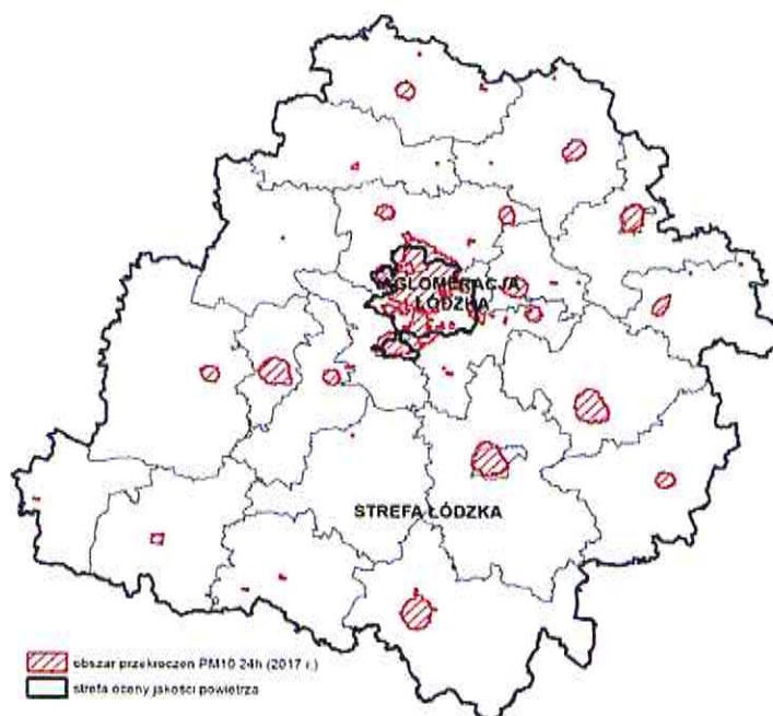
Mapa 8. Obszary przekroczeń średniej 24-godzinnej wartości poziomu dopuszczalnego pyłu PM10 w 2017r.
